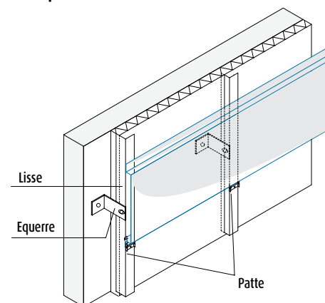
Composants associés pour ossature métallique
